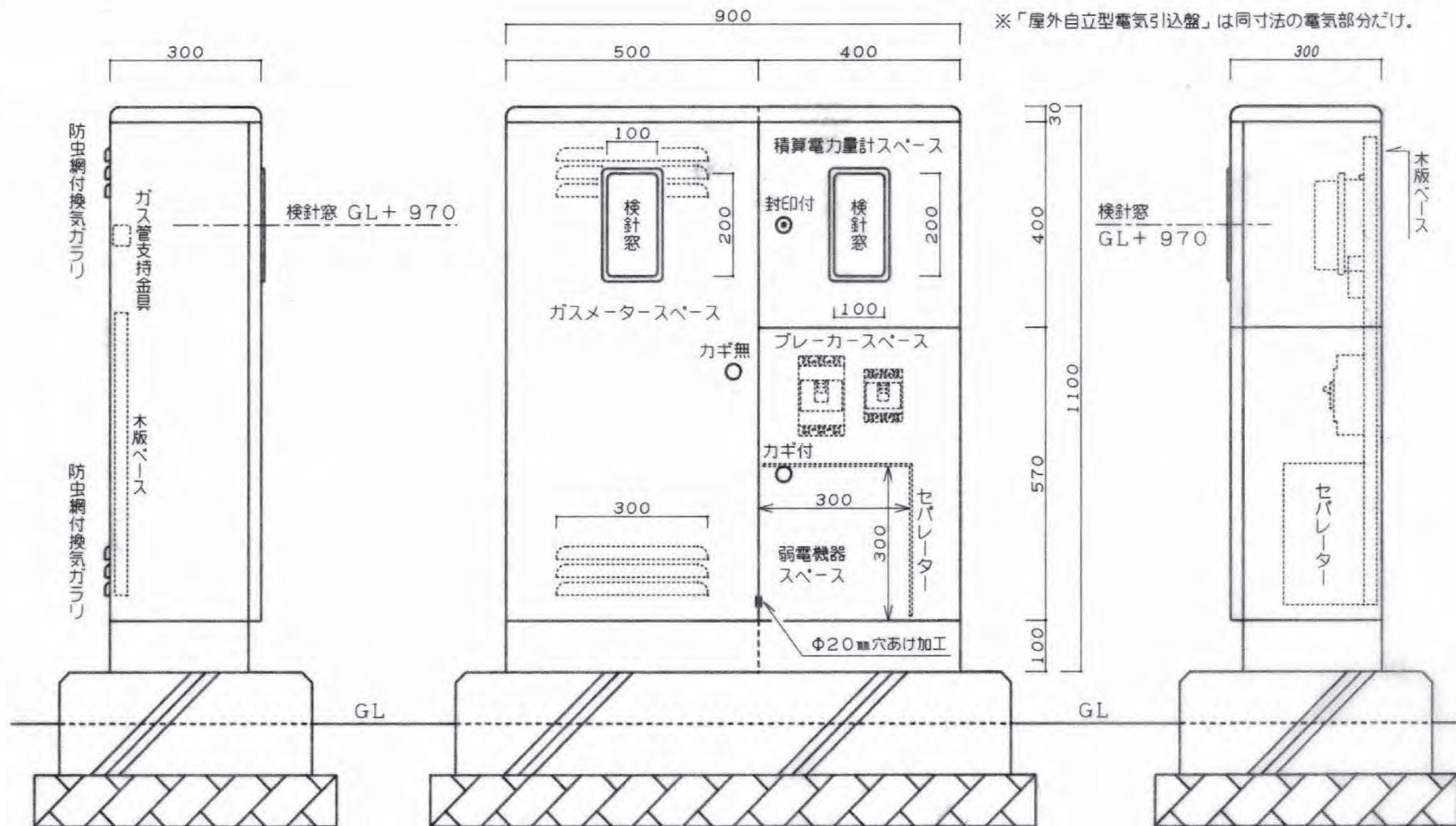
屋外自立型引込盤姿図 (S=1/10)
